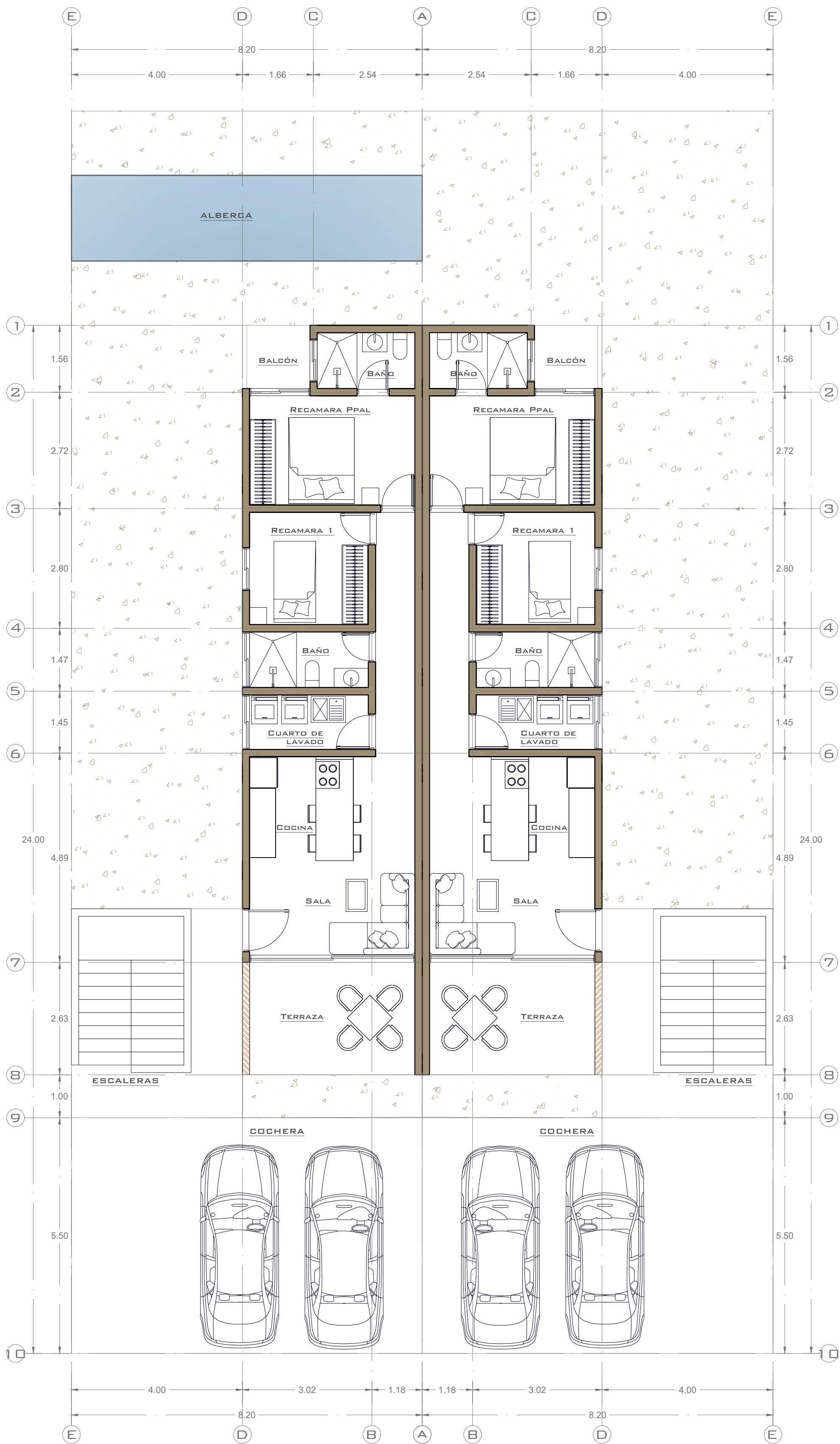
PLANTA ARQUITECTÓNICA
