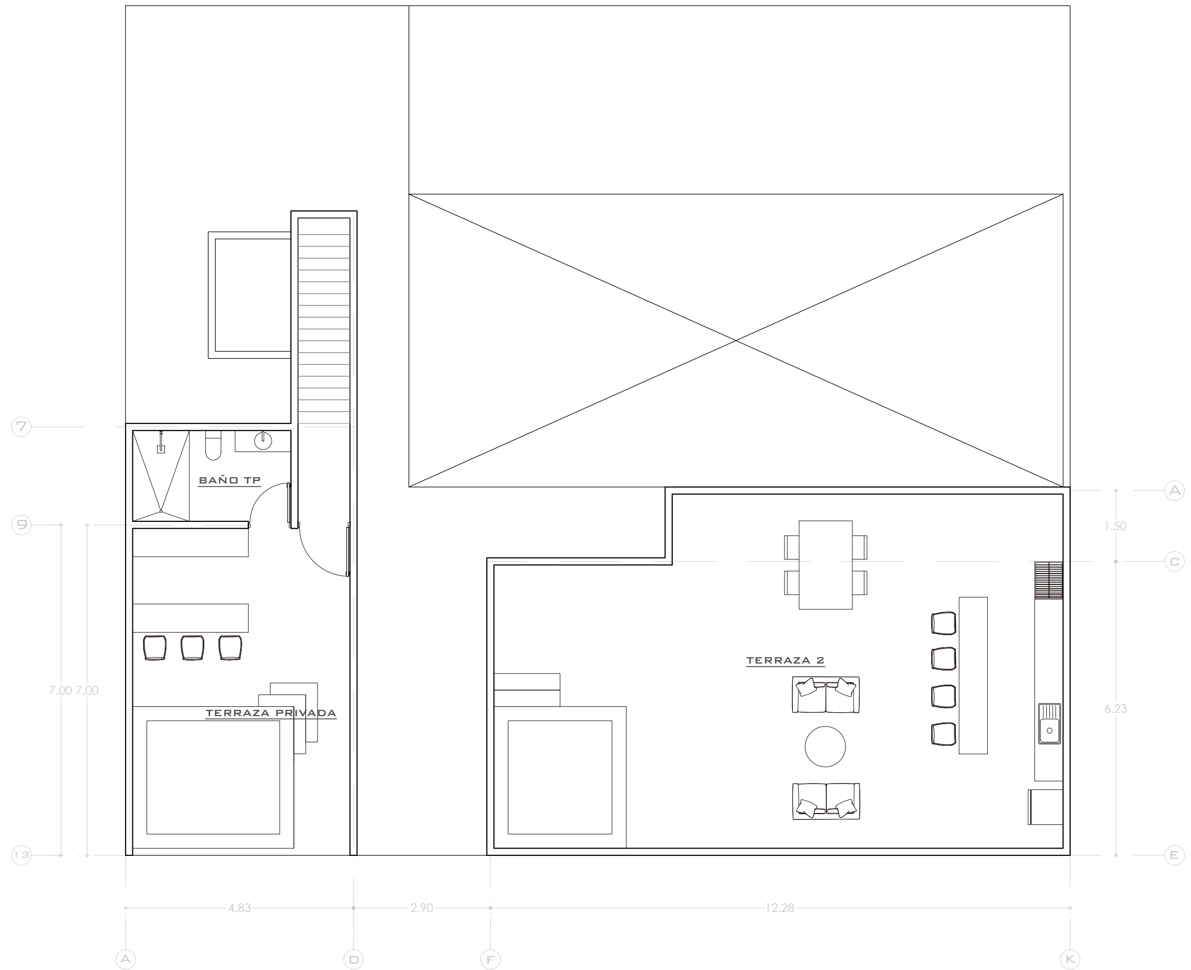
PLANTA ARQUITECTÓNICA TERRAZA
