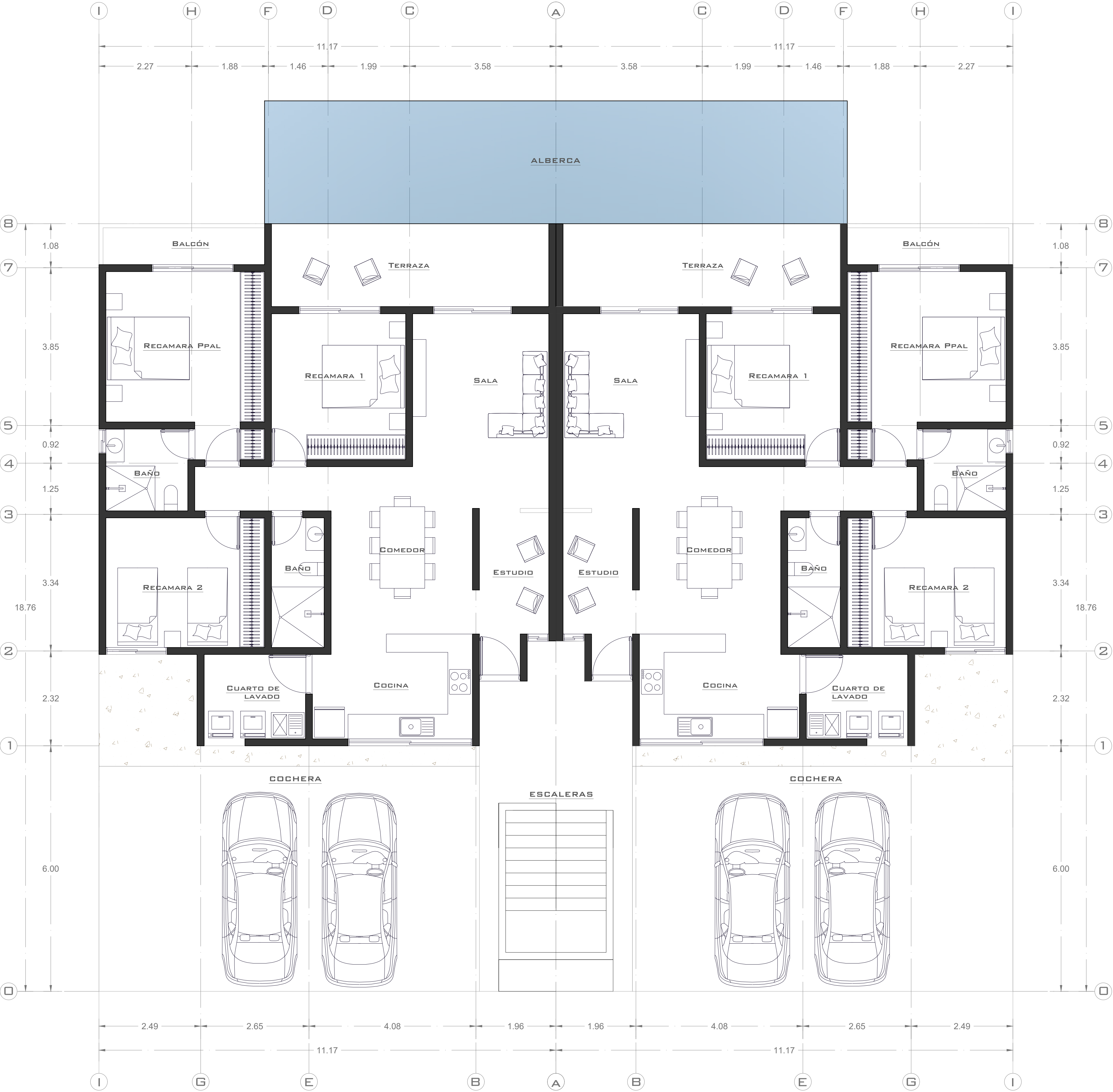
PLANTA ARQUITECTÓNICA
